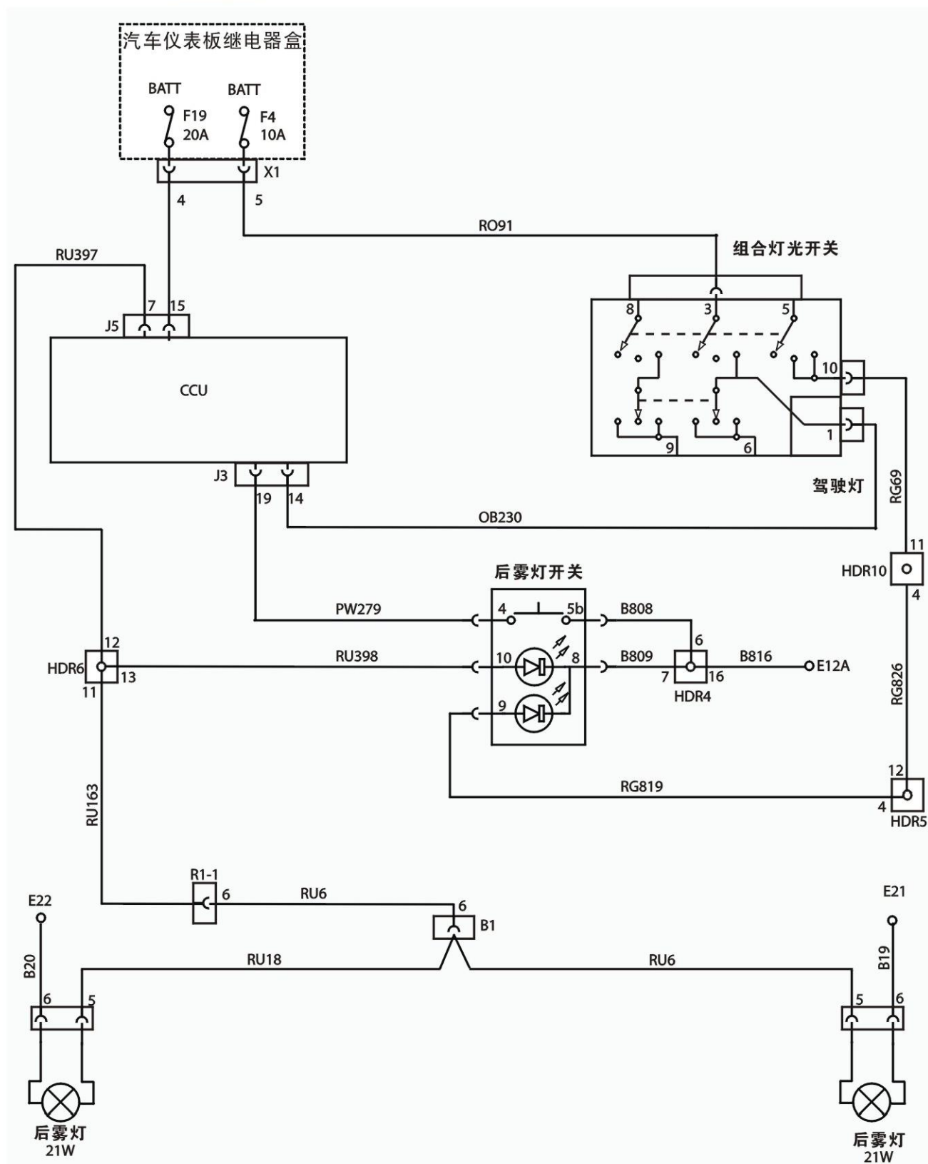
后雾灯电路
